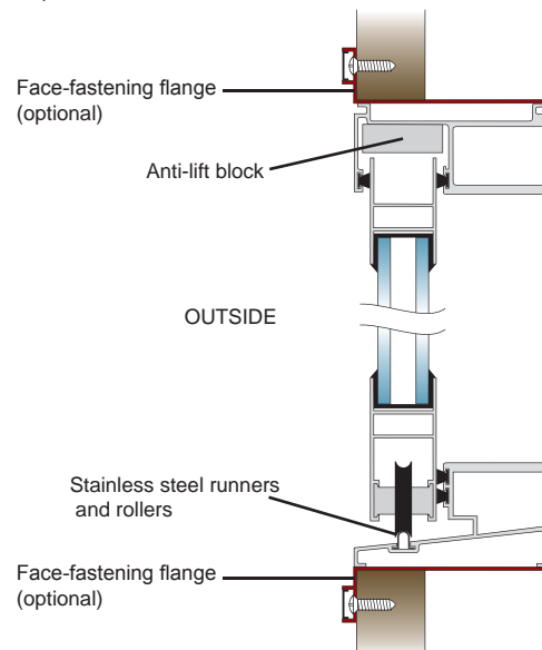
Cranked patio door
